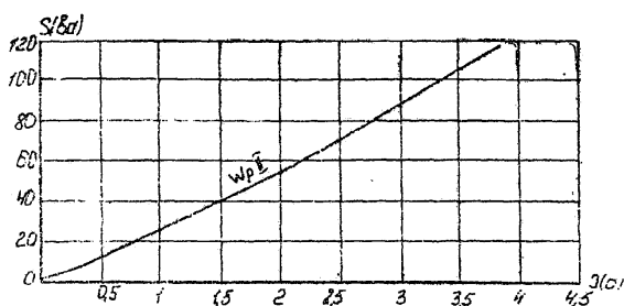
Черт. 19. Мощность, потребляемая обмоткой реле типа ДЗТ-11/3 в аварийном режиме.
