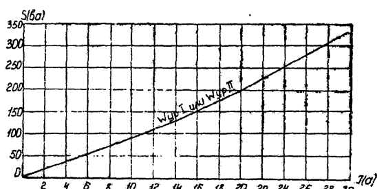
Черт. 17. Мощность, потребляемая обмоткой реле типа ДЗТ-11/2 в аварийном режиме.
