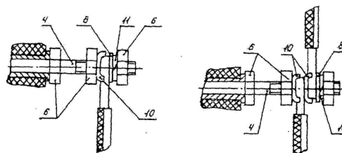
б) для заднего присоединения шпилькой
