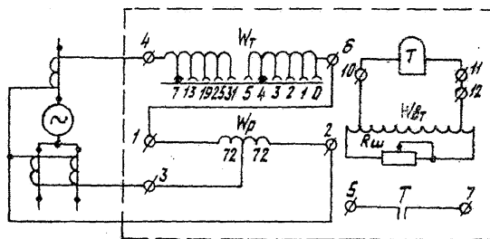
Черт. 7. Принципиальная схема реле типа ДЗТ-11/5 и схема его включения для генератора с двумя выводами на фазу к нейтрали.
