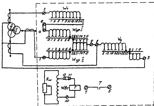
Черт. 3. Принципиальная схема реле типа ДЗТ-11 и схема его включения.
