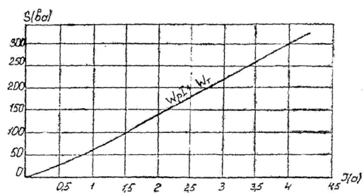
Черт. 21. Мощность, потребляемая обмоткой реле типа ДЗТ-11/4 в аварийном режиме.
