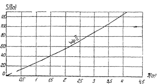
Черт. 22. Мощность, потребляемая обмоткой реле типа ДЗТ-11/4 в аварийном режиме.
