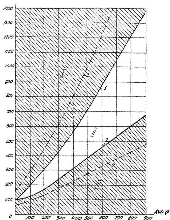
Черт. 9. Тормозные характеристики реле I – Зона срабатывания. II – Зона срабатывания или торможения в зависимости от угла между тормозным и рабочим токами. III – Зона торможения.
