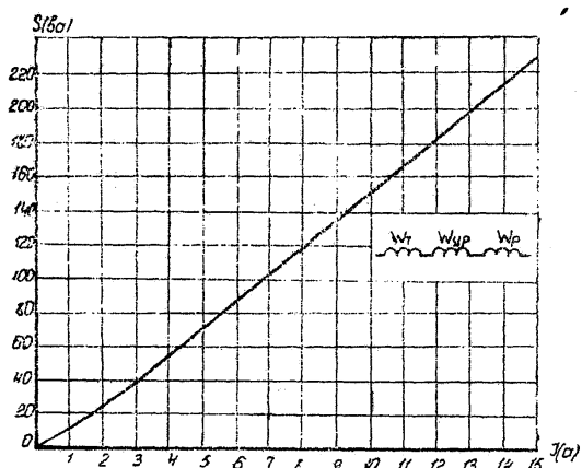
Черт. 15. Мощность, потребляемая в аварийном режиме обмоткой реле типа ДЗТ-11.
