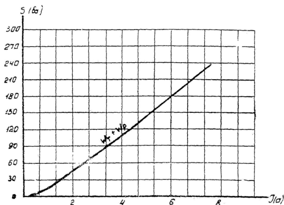
Черт. 24. Мощность, потребляемая обмоткой реле типа ДЗТ-11/5 в аварийном режиме.
