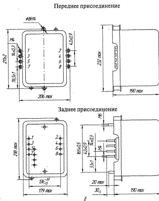
Черт. 8. Габаритные, установочные и присоединительные размеры реле. Размеры без предельных отклонений – максимальные.
