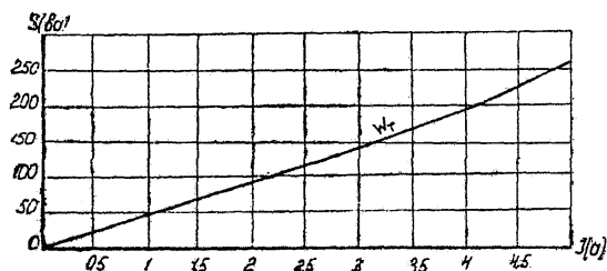
Черт. 13. Мощность, потребляемая обмоткой реле типа ДЗТ-11/4 в нормальном режиме.
