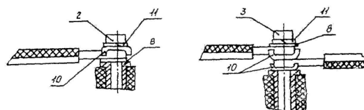
в) для заднего присоединения винтом
