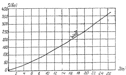
Черт. 23. Мощность, потребляемая обмоткой реле типа ДЗТ-11/4 в аварийном режиме.
