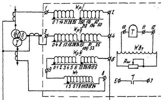
Черт. 2. Схема расположения обмоток реле типов ДЗТ-11, ДЗТ-11/2, ДЗТ-11/3, ДЗТ-11/4, ДЗТ-11/5 на магнитопроводе НТТ.
